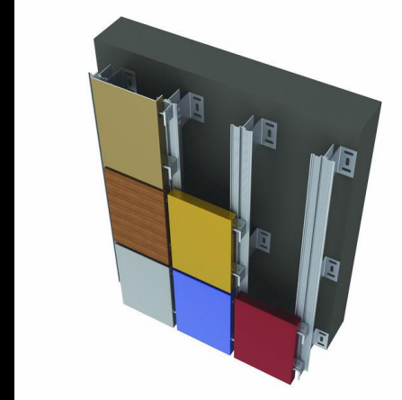
صفائح مغلطنة tôles galvanisées
