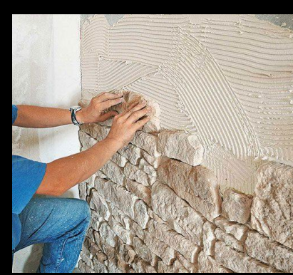
Habillage en parement depierre/
